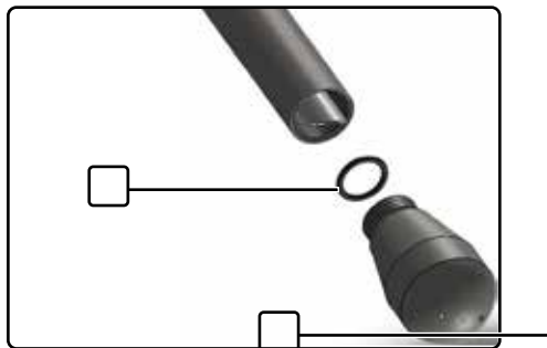
Ilus. 10 boquilla del tubo de vapor, desmontada
